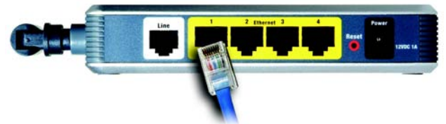
Abbildung 4-2: Anschließen eines Computers
